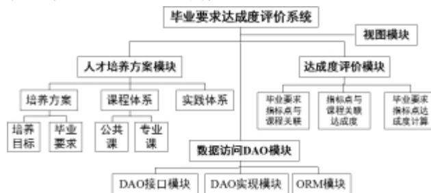
图 1 毕业要求达成度评价系统模块结构
